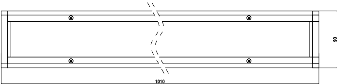
cutout size:L 1005*W80*H100mm±1mm
